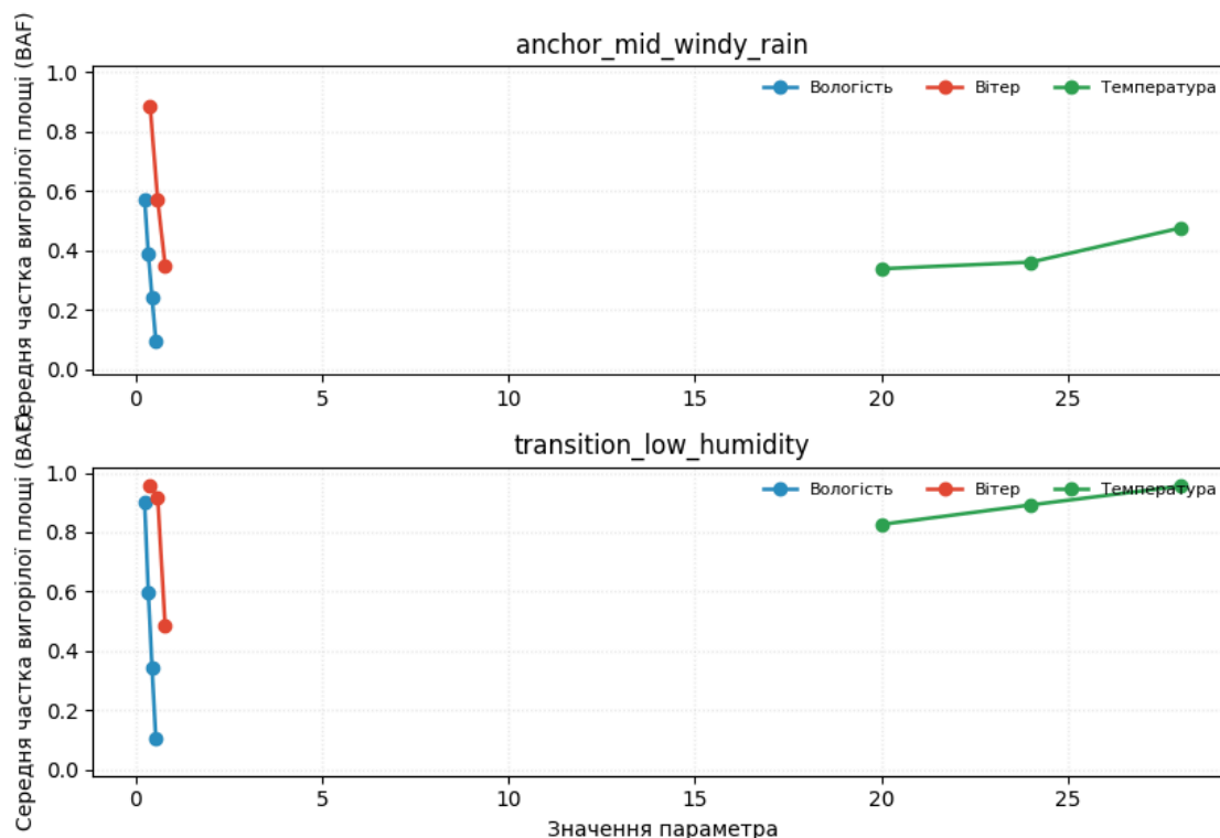
Рис. 4.2.1 – Криві однофакторної чутливості середньої частки вигорілої площі до зміни вологості, температури та сили вітру
