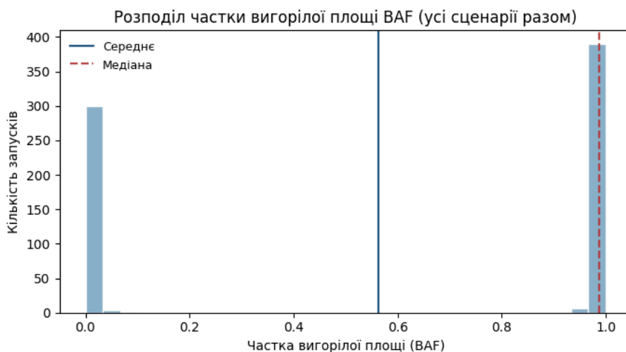
Рис. 4.1.1 – Розподіл частки вигорілої площі BAF по всіх базових сценаріях
